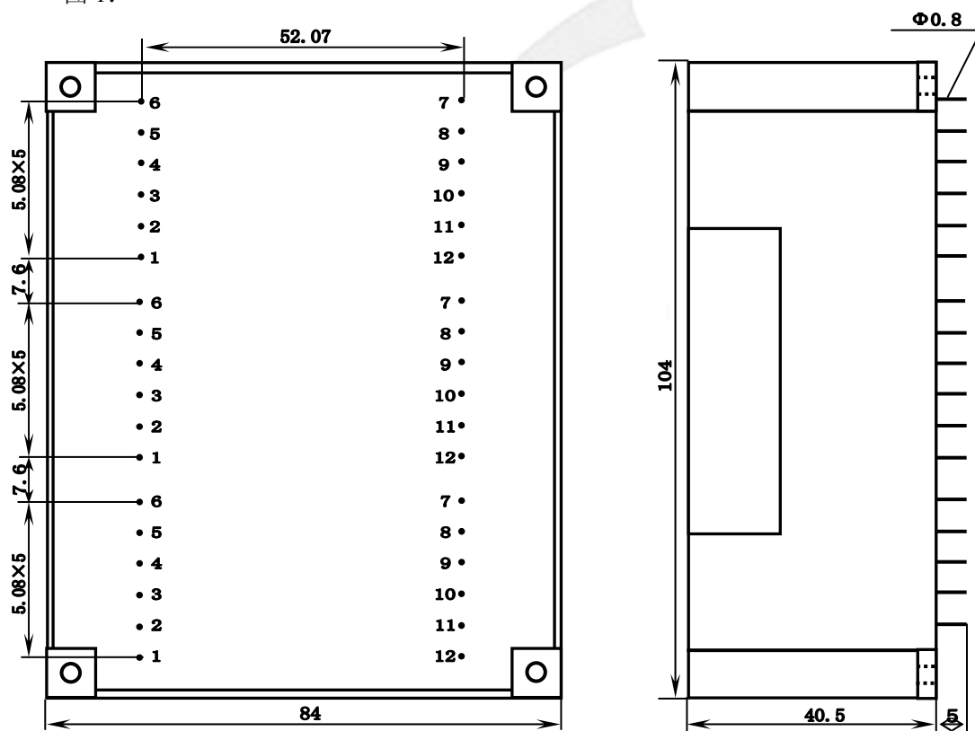
外形背视图
